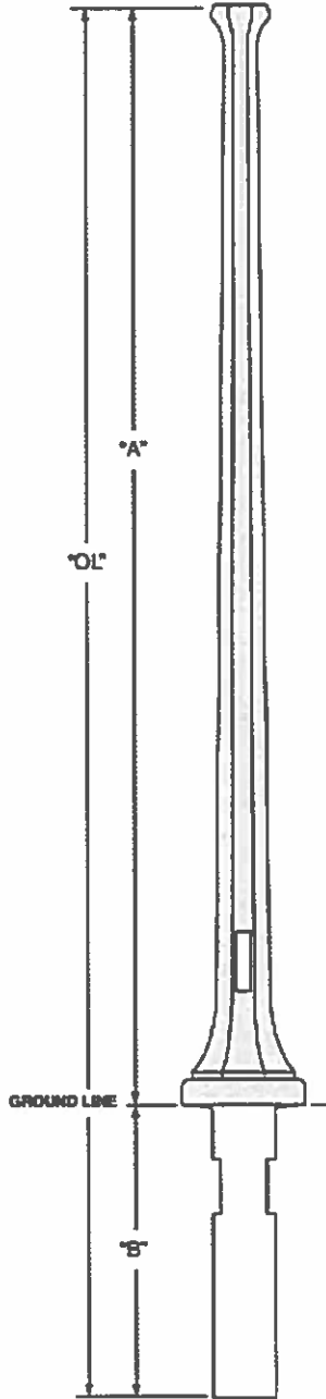
Ameron Centrecon VEM-4.6
